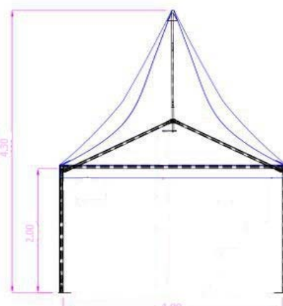
Chapiteau 4x4
