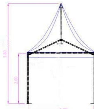
Chapiteau 3x3
